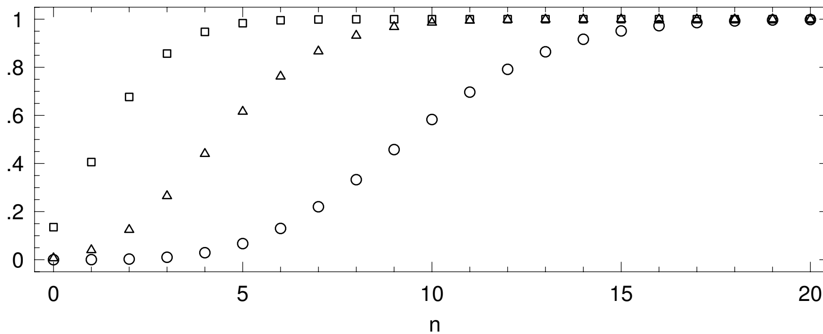
F(n, \langle n \rangle) , Poisson CDF
